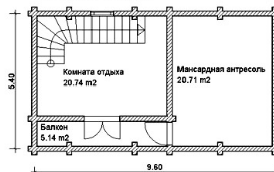
План мансарды
