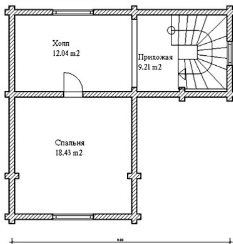
ПЛАН МАНСАРДЫ
