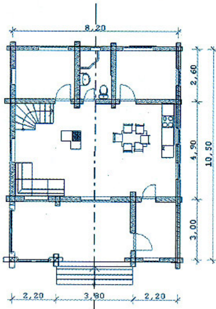
План 1 этажа
