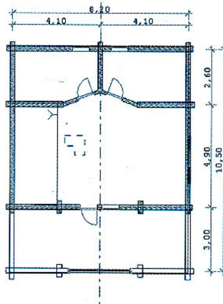
План 2 этажа
