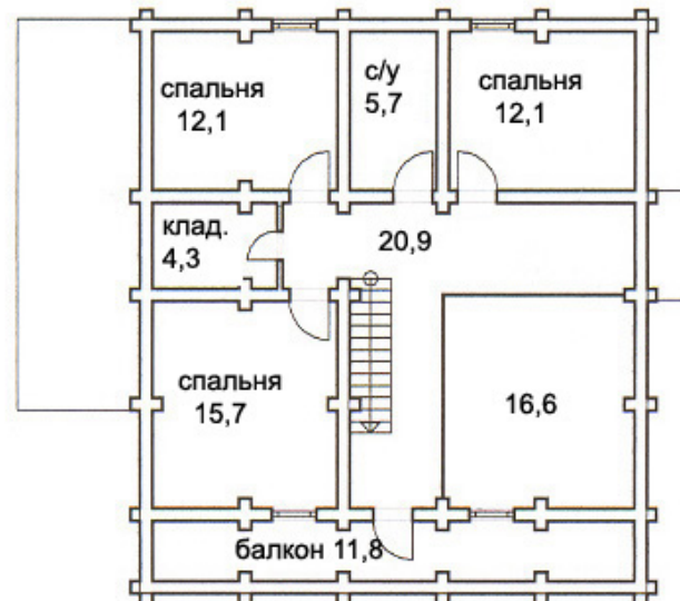
План мансарды
