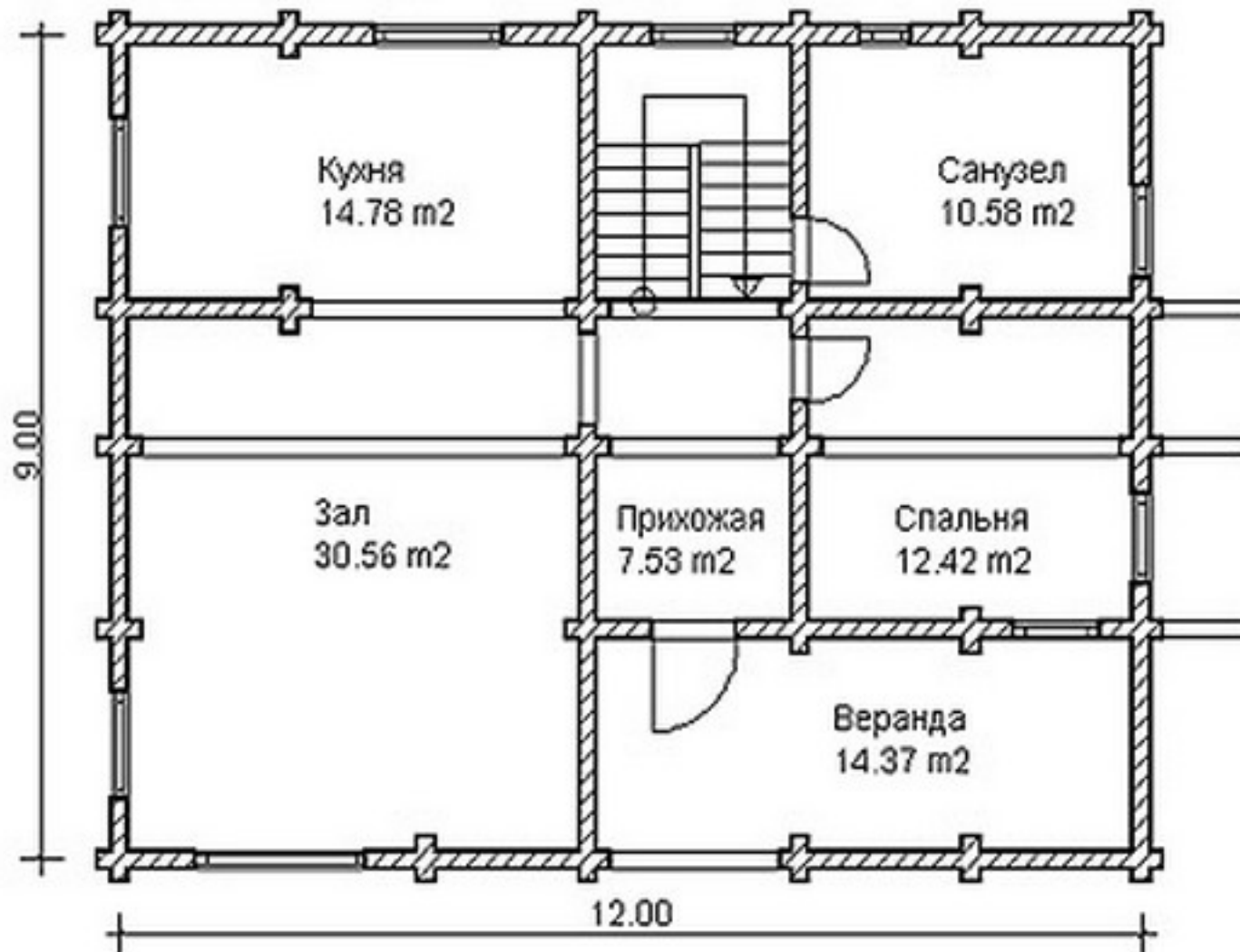
План 1 этажа
