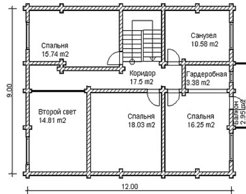
План 2 этажа
