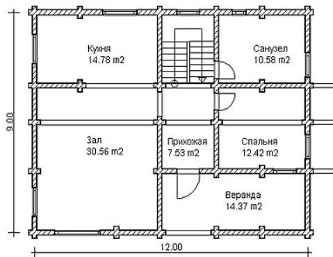
План 1 этажа
