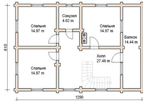
План 2 этажа
