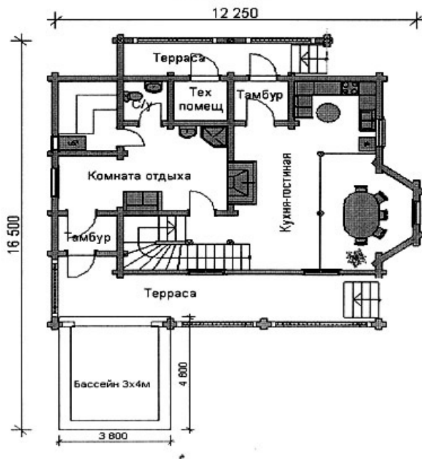
План 1 этажа
